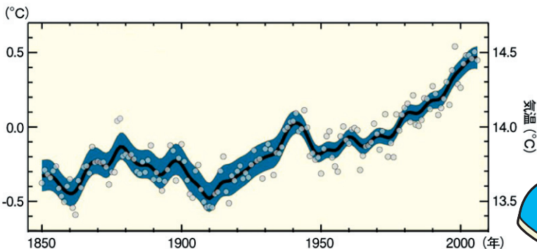
世界平均気温の変化
