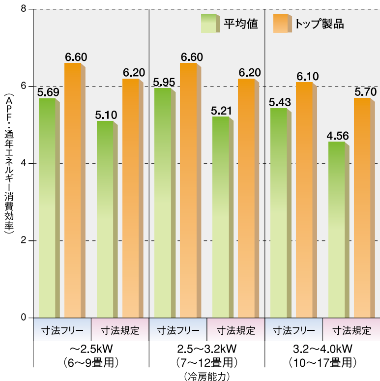
図3 エアコンの冷房能力別APFの比較
