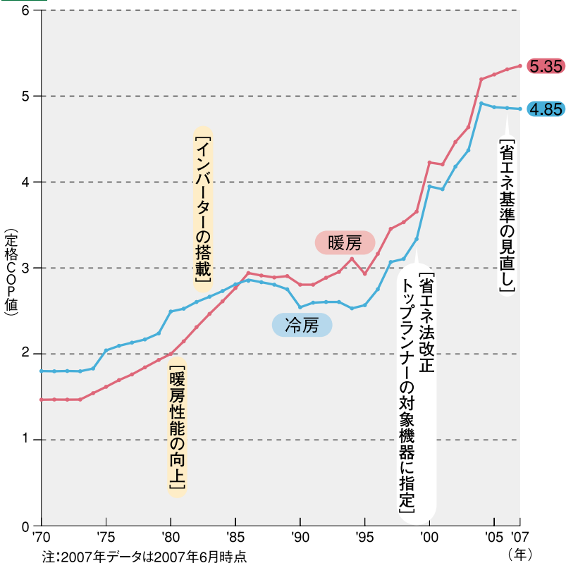
図2 フロー（販売）ベースの冷暖房COPの推移
