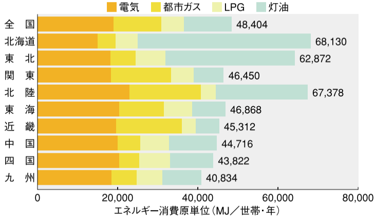
図5 世帯あたり燃料種別エネルギー消費原単位の地域比較(2005年)
