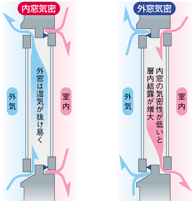
図7 内窓と外窓の気密バランス
