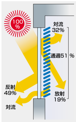
3ミリガラス+内側ブラインド
