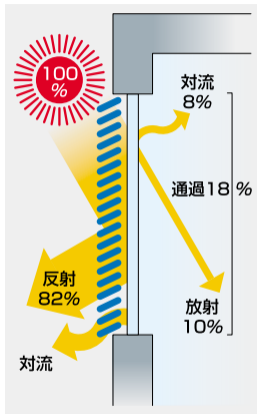
3ミリガラス+外側ブラインド
